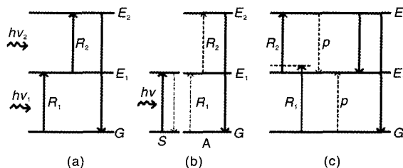
图 1 上转换机制示意图：(a) 激发态吸收，(b) 能量传递，(c) 光子雪崩
